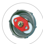
Réducteur à satellites et planétaire
